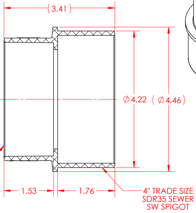
SECTION A-A
