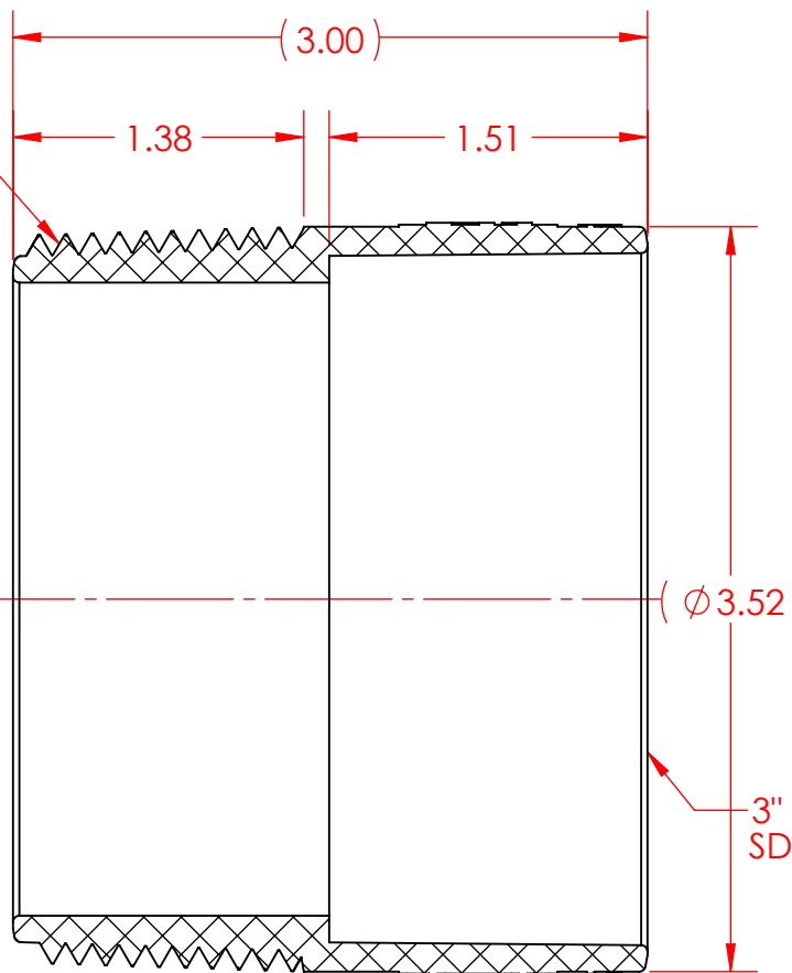
SECTION A-A
